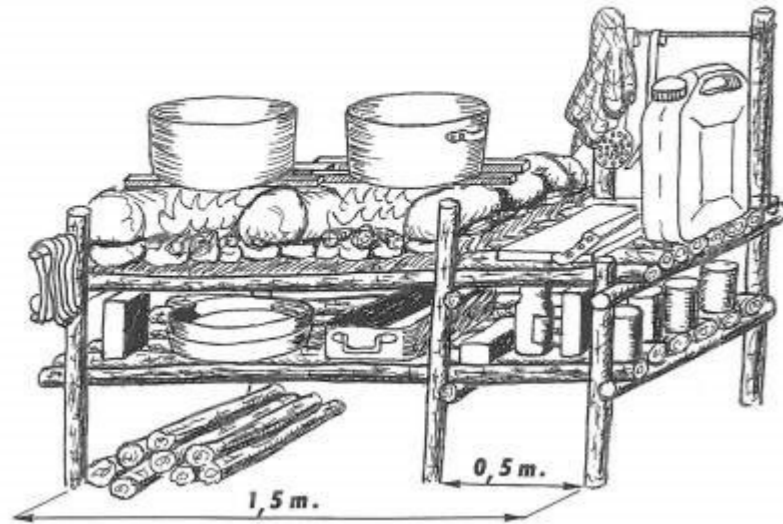
EXEMPLE DE TABLE A FEU EN BOIS.
