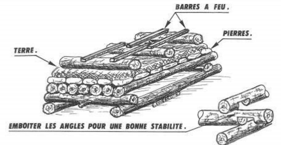
MIXTE: BOIS ET PIERRES.
